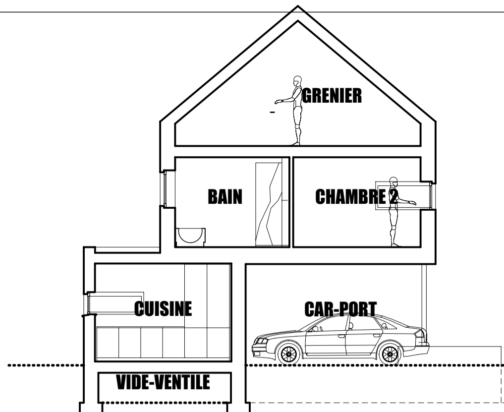
COUPE AA
