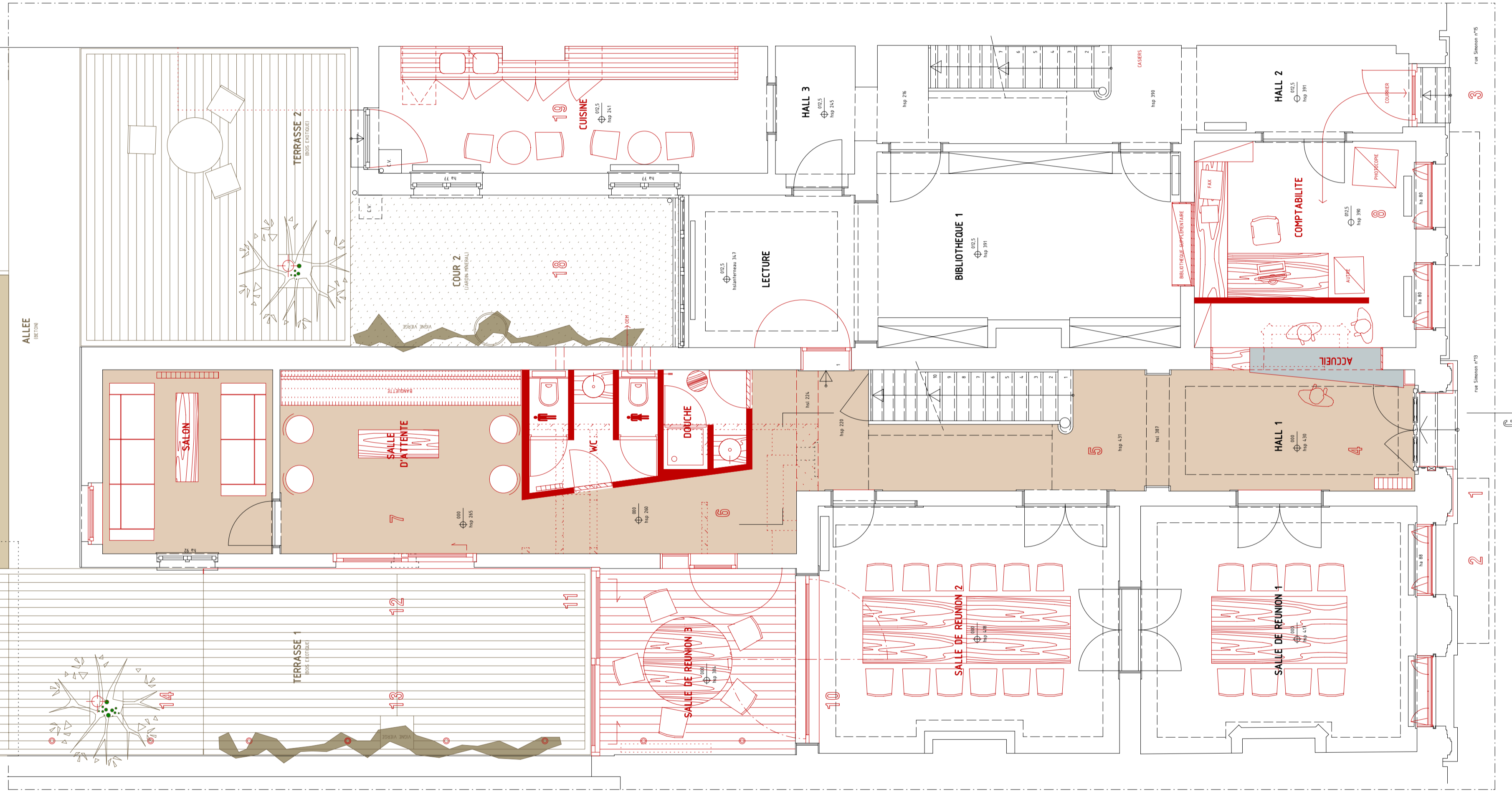
REZ DE CHAUSSEE PROJETE
