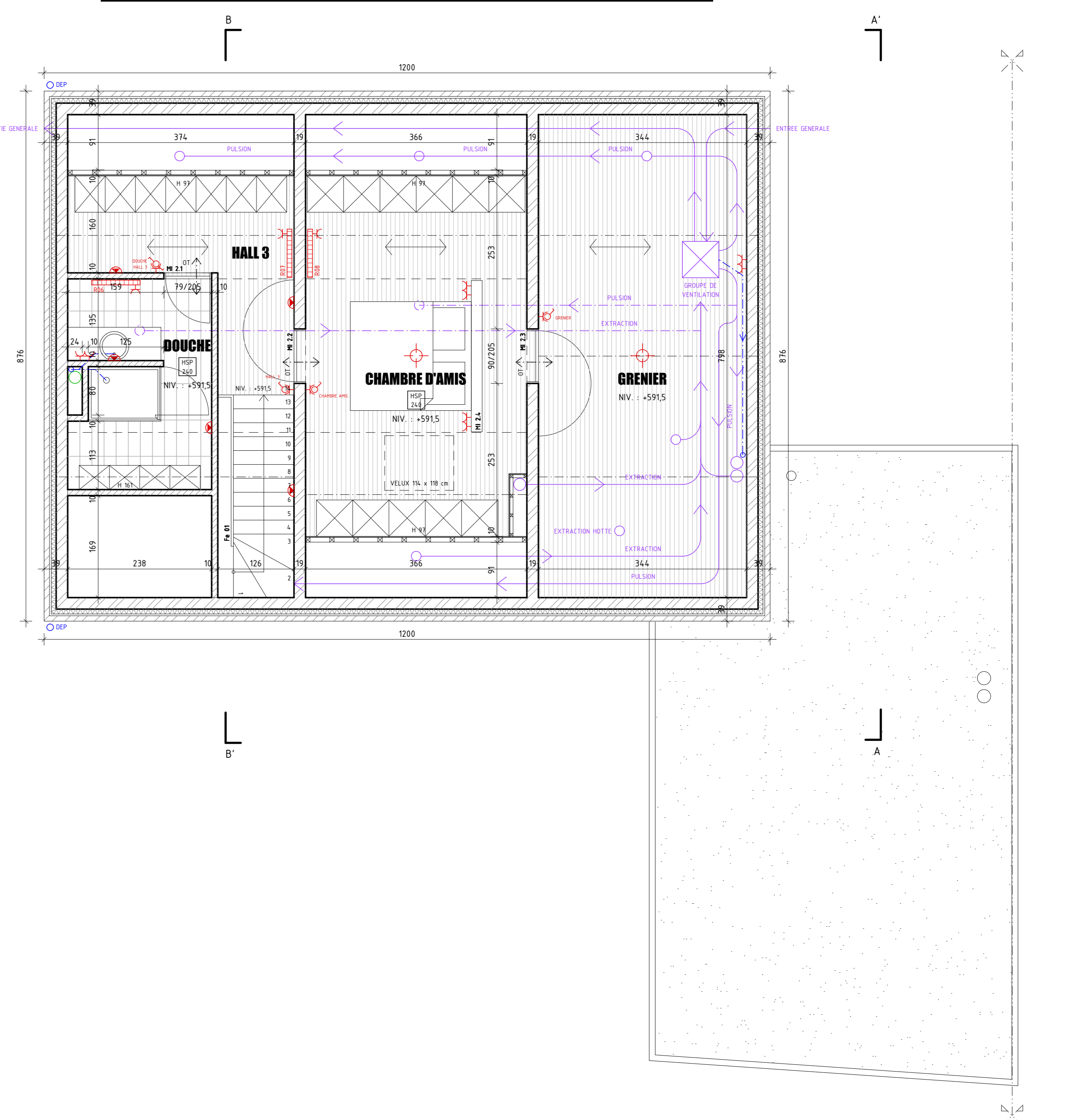
VUE EN PLAN ETAGE 2 - NIV. : + 591,5
