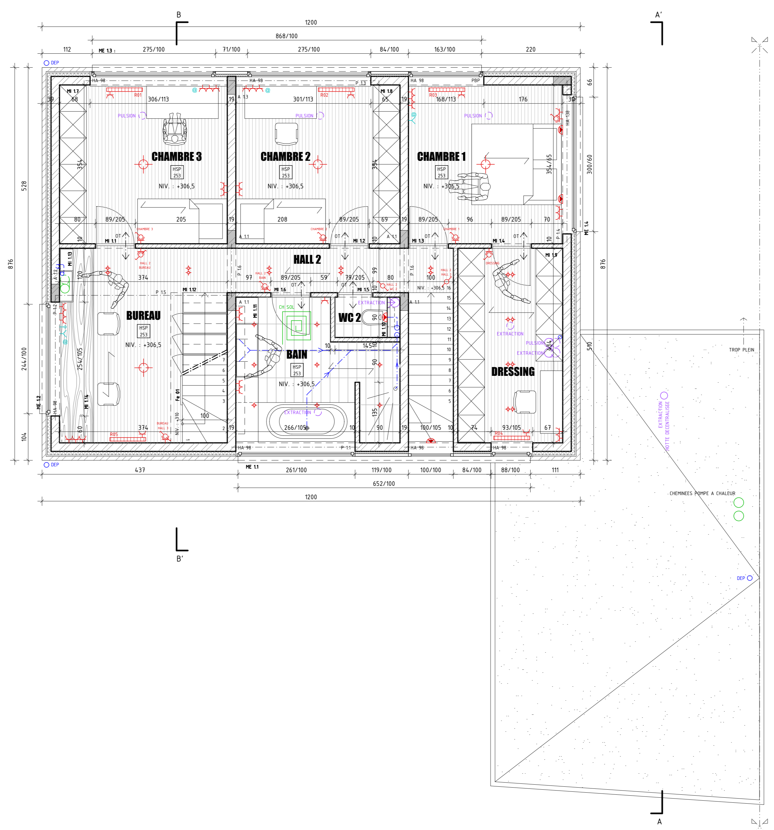
VUE EN PLAN ETAGE 1 - NIV. : + 306,5
