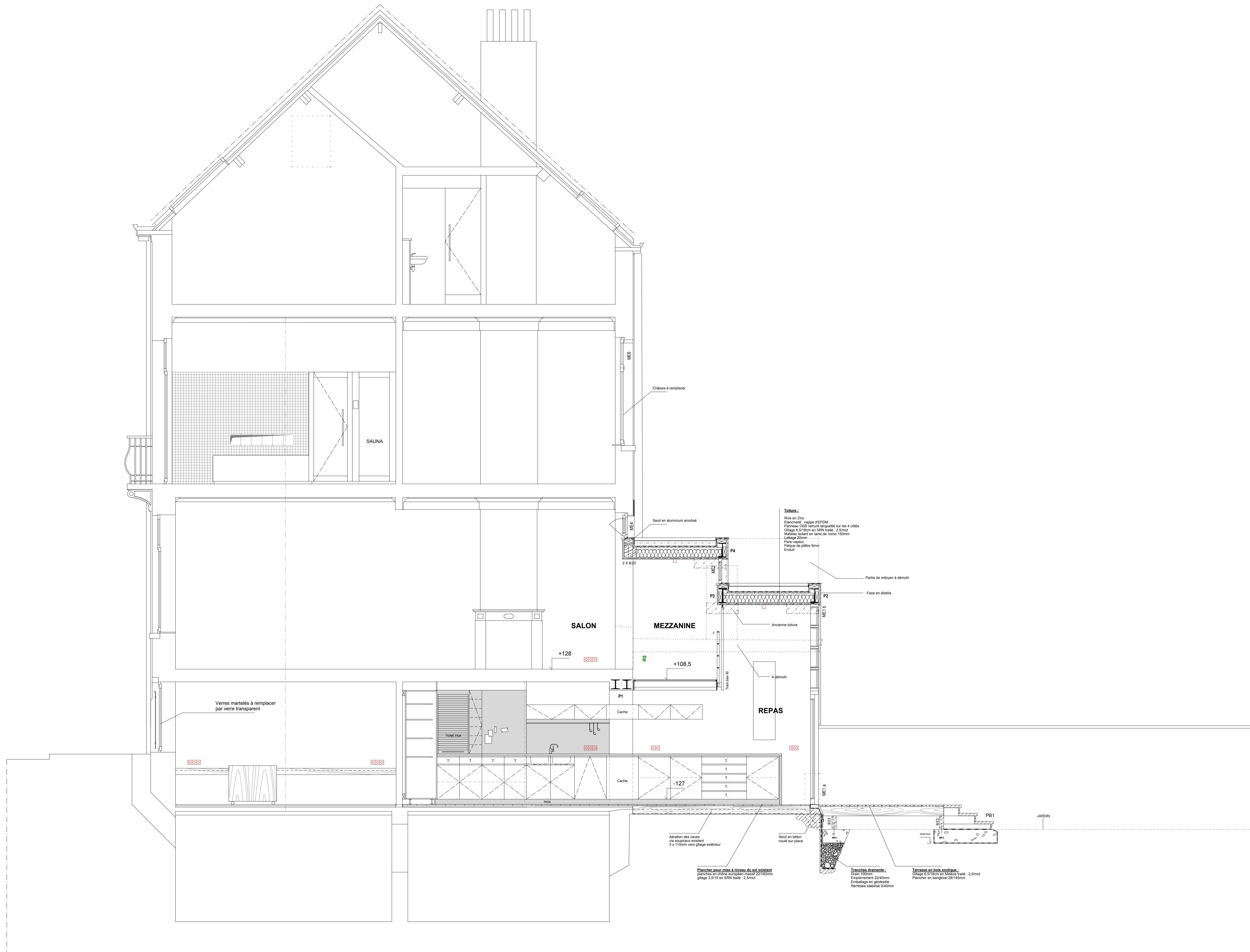
COUPE LONGITUDINALE AA
