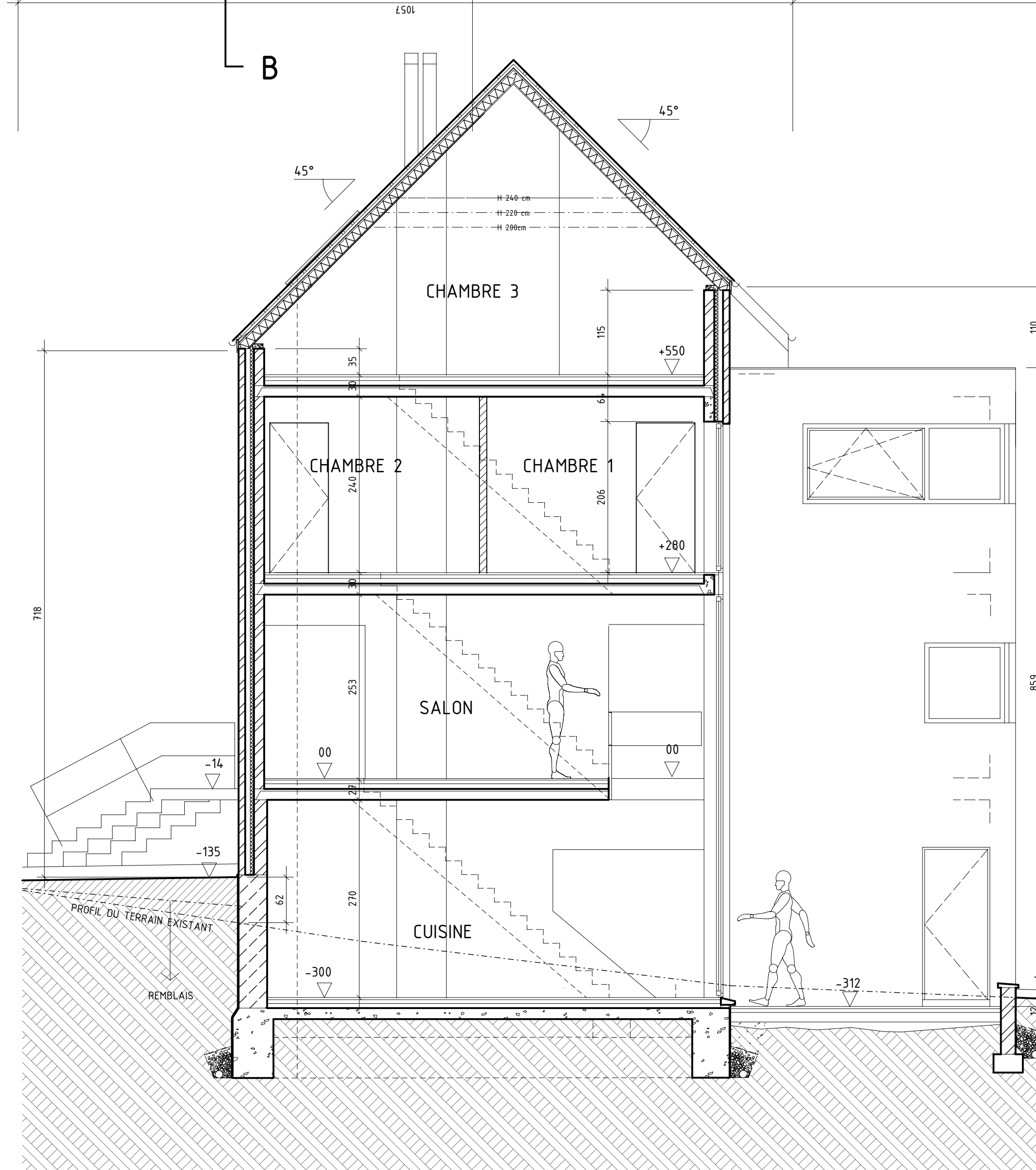
Coupe AA
