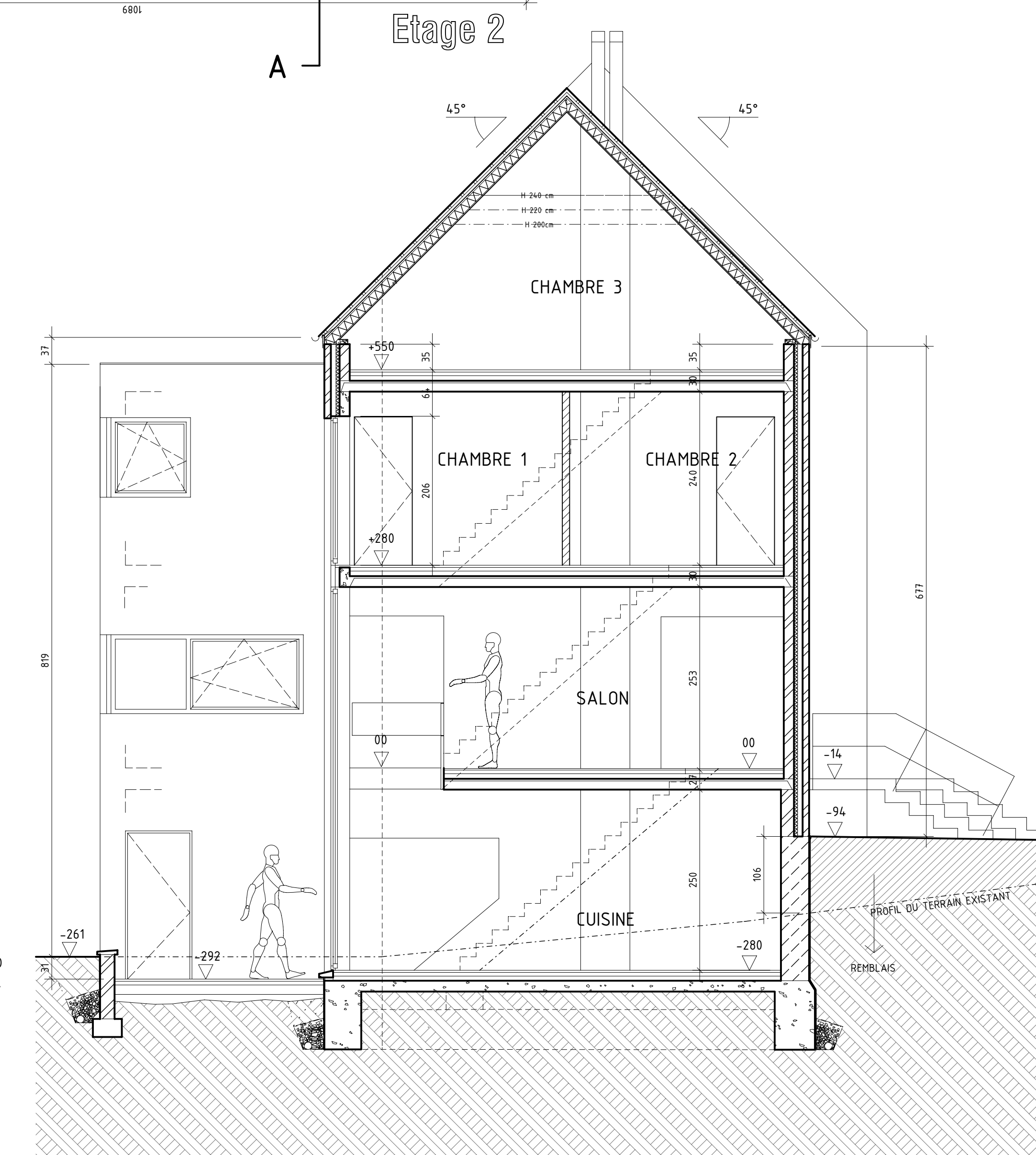
Coupe BB
